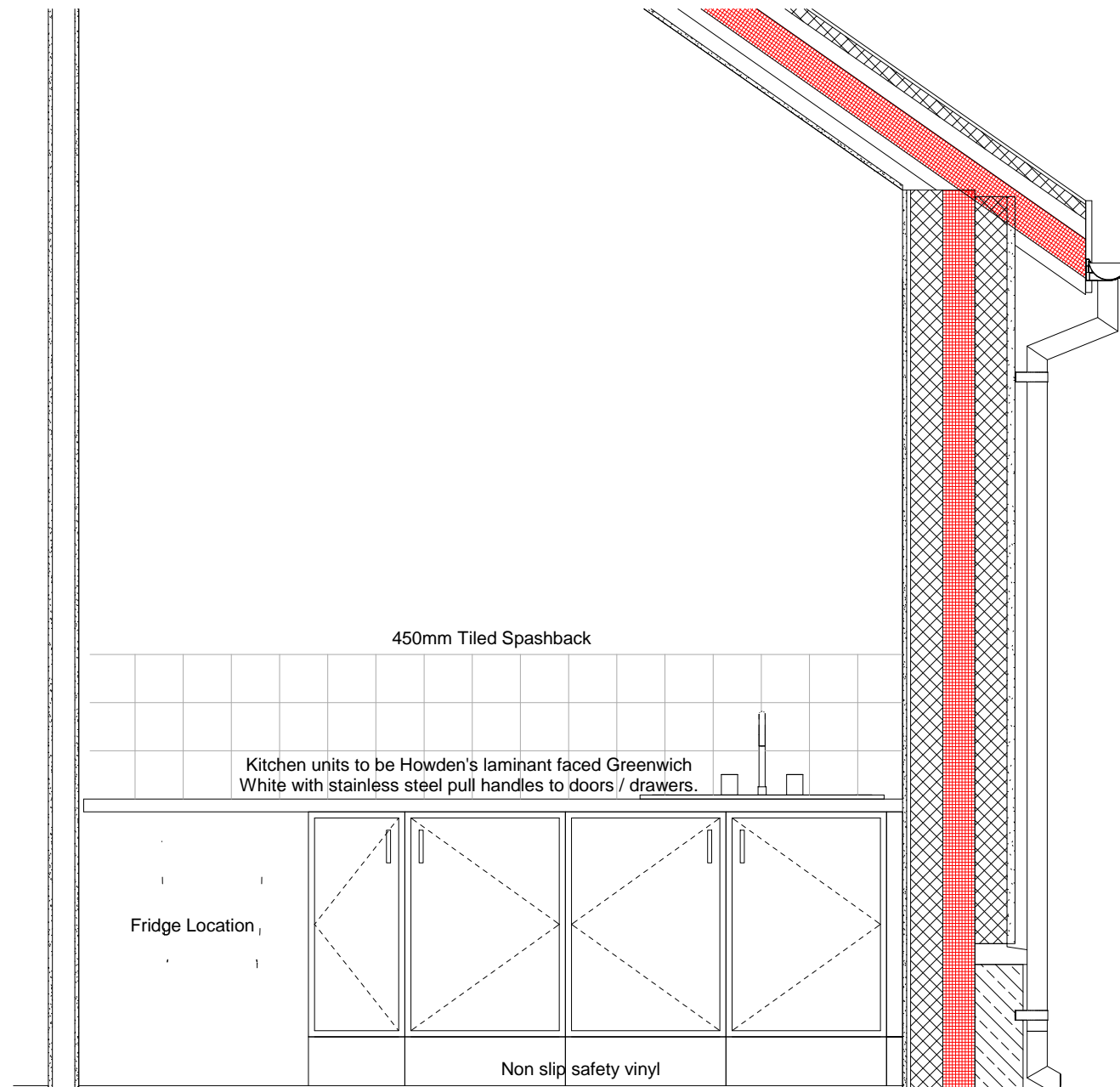
Elevation A 1 : 10
